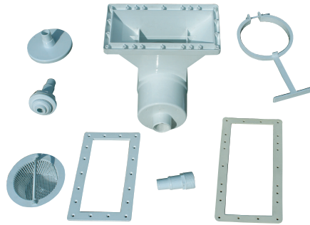
Wide Angle Skimmer – ENS110
