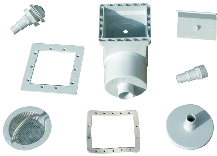
Standard Skimmer – ENS100
