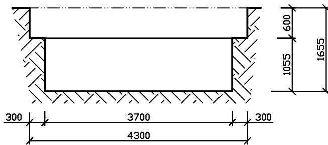
ŘEZ B-B
